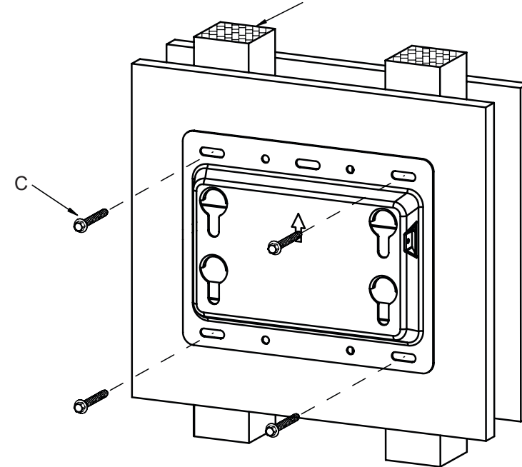
Stud walls
